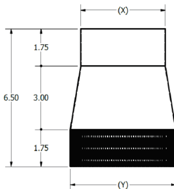
Réduit femelle aux deux embouts
